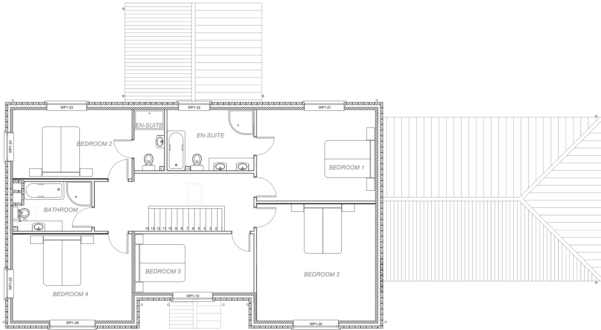
1:75 @ A1
